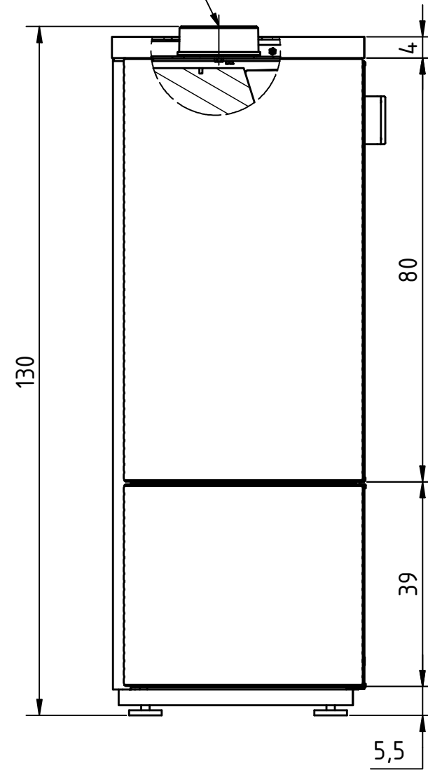
Rauchrohranschluss Ø15 Seite
